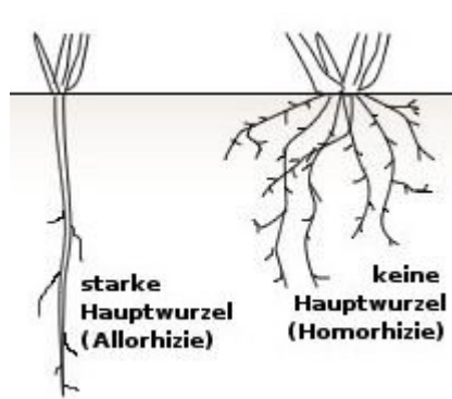
Abbildung 6: Wurzelsysteme 131
